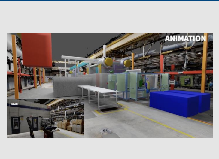
Green- & Brownfield Planungen – Scan, Modellierung und AR-Erlebnis
