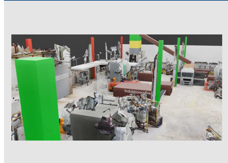
Plausibilisieren von Planungsständen – Analyse am Digitalen Planungszwilling
